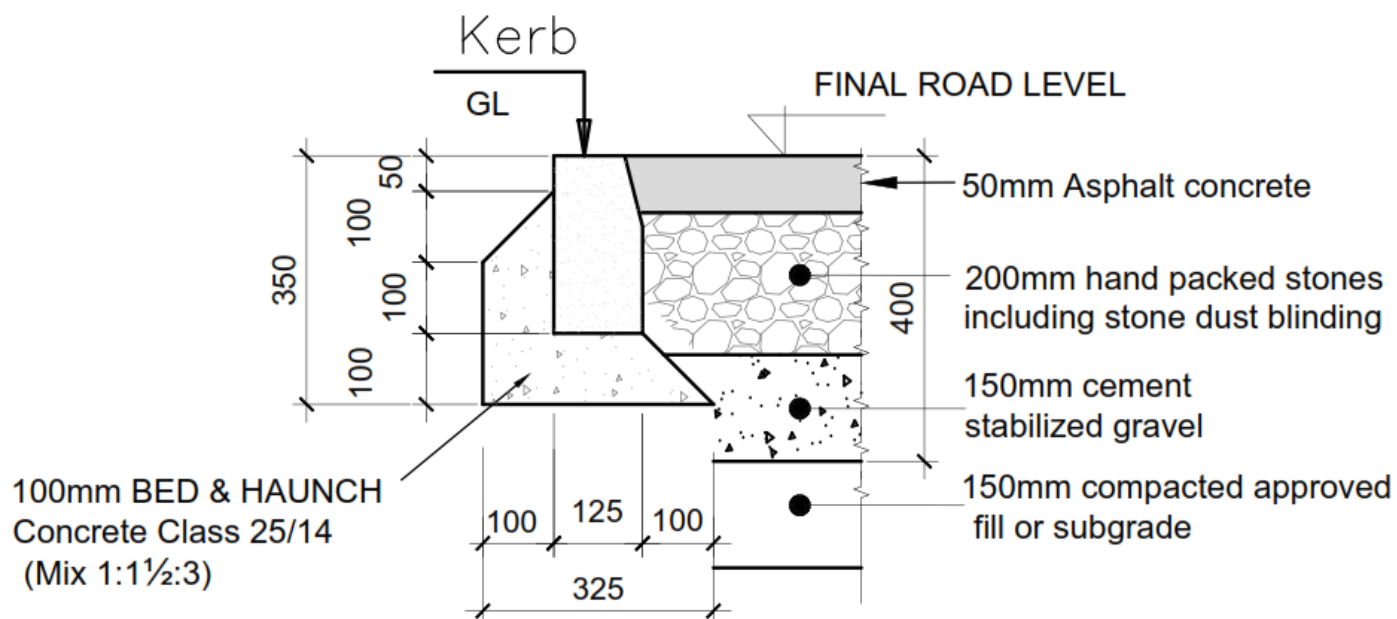
125X250mm KERB.-FIG K3
